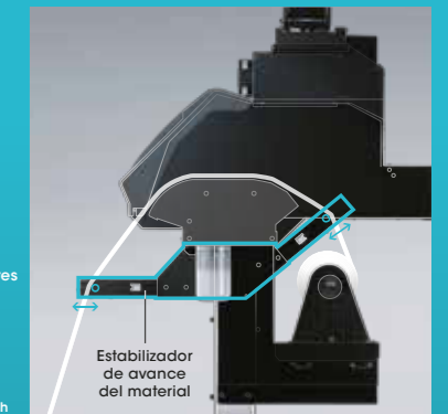
Imagen del estabilizador de avance del material
